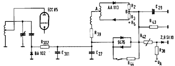
Prinzipschaltung der autom. UKW-Scharfabbstimmung
