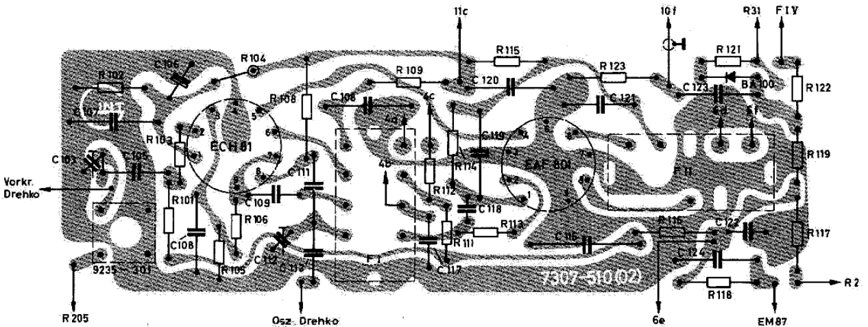
Druckschaltungsplatte 460 kHz auf die Lötseite gesehen
