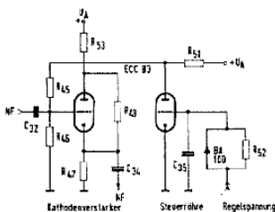
Prinzipschaltung der Stillabbstimmung
